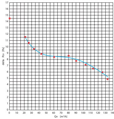
Fan efficiency characteristic Rohrlüfterleistungskennlinie
